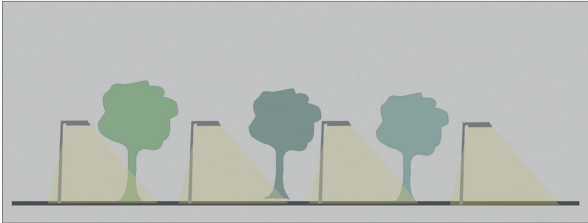
Abbildung 6: Beispiel für abgeschirmte Leuchten auf kurzen Masten zur Verhinderung von Lichtimmissionen in benachbarte Jagdhabitats, Quelle: H. LIMPENS IN EUROBATS, 2019.
